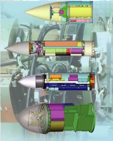
飛彈尋標器
